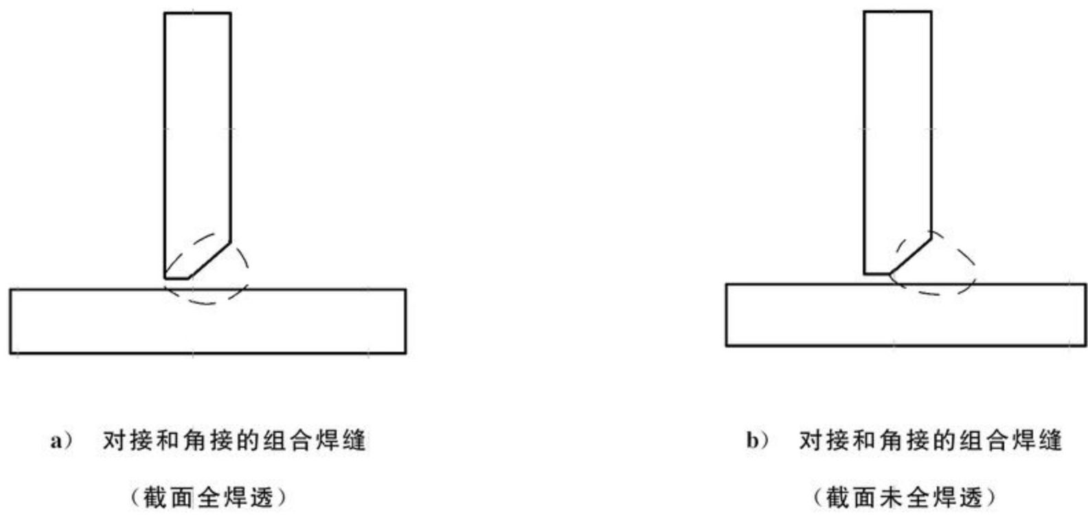
图 F.2 T形接头组合焊缝
