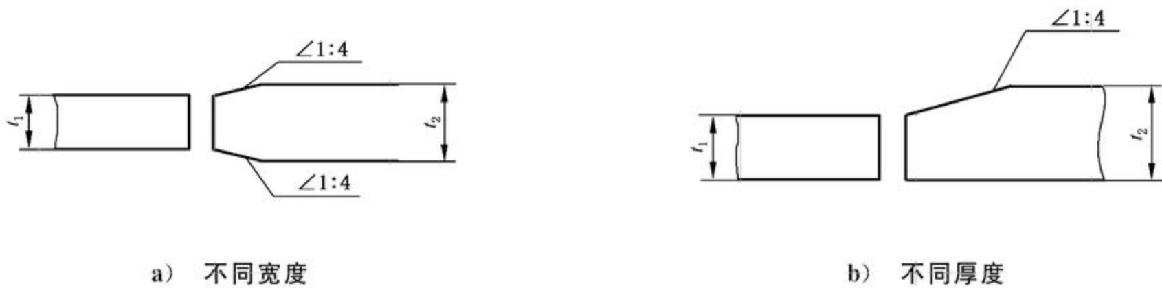
图 7 不同宽度或厚度钢板的拼接
