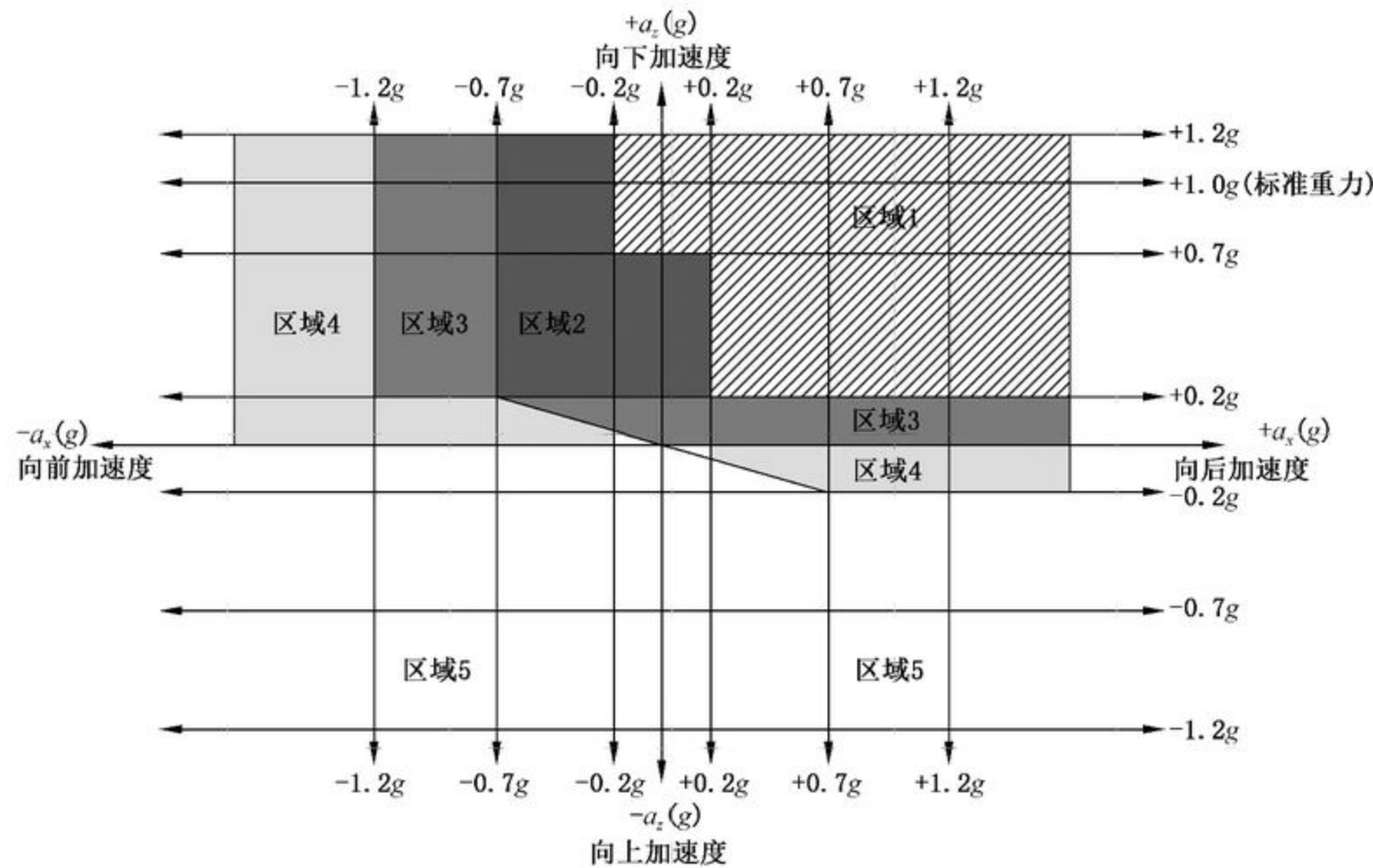
图 8 设计加速度的 5 个区域
