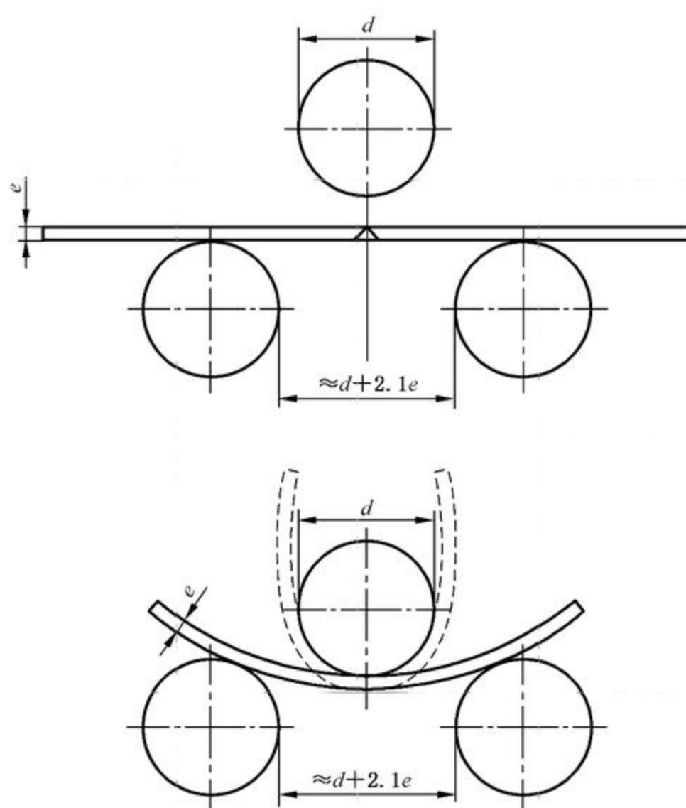
图 7 对接接头弯曲试验
