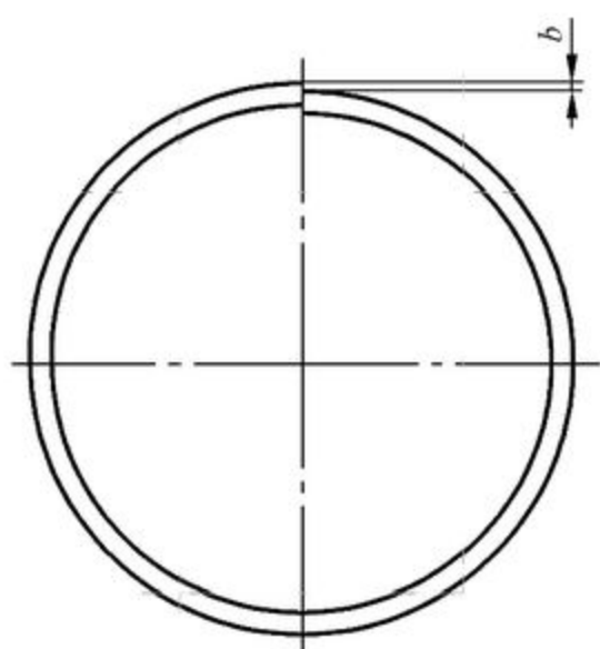
图3 筒体纵焊缝对口错边量
