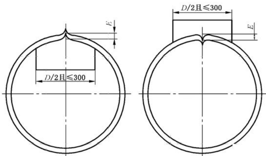
图4 筒体纵焊缝棱角高度
