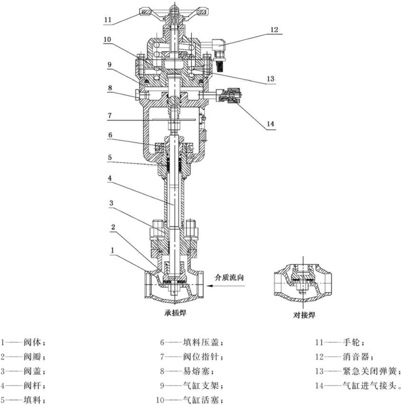
图 1 焊接式低温紧急切断阀
