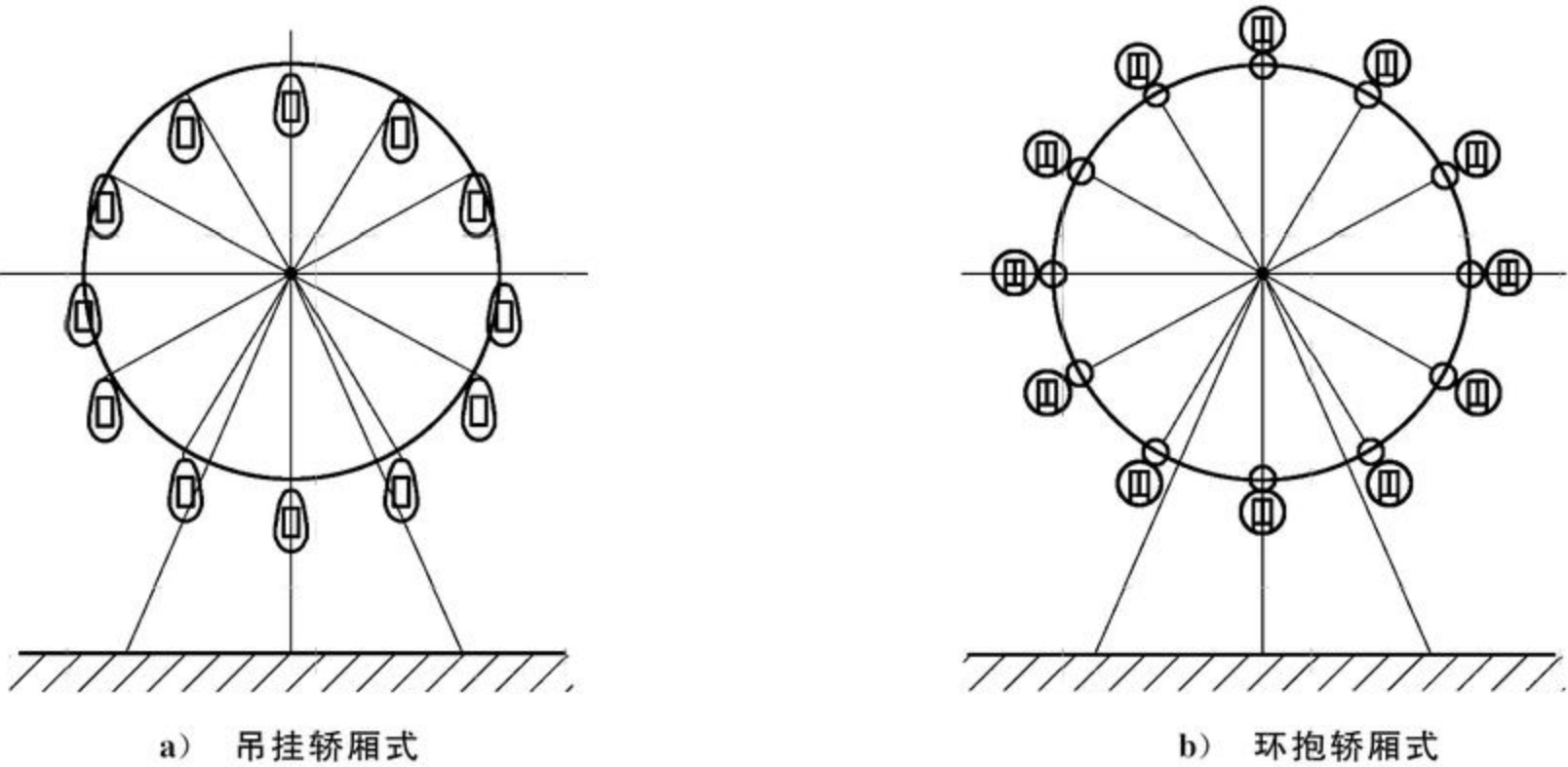
图 A.1 有主轴摩天轮型(A 型)
