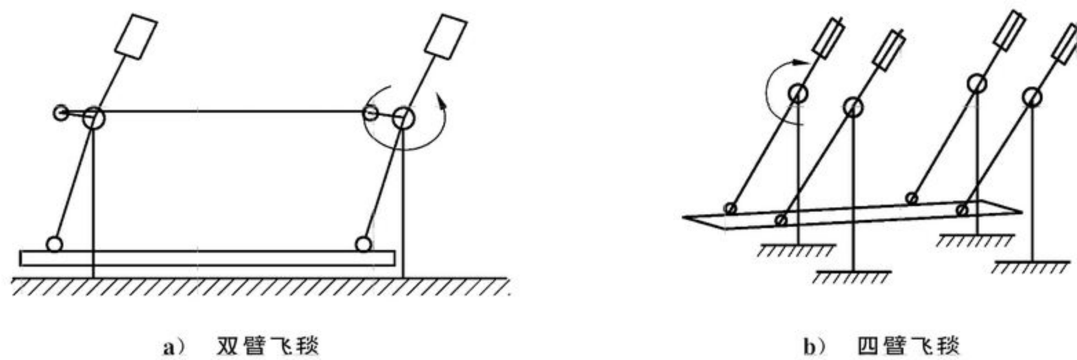
图 A.6 飞毯型(F 型)
