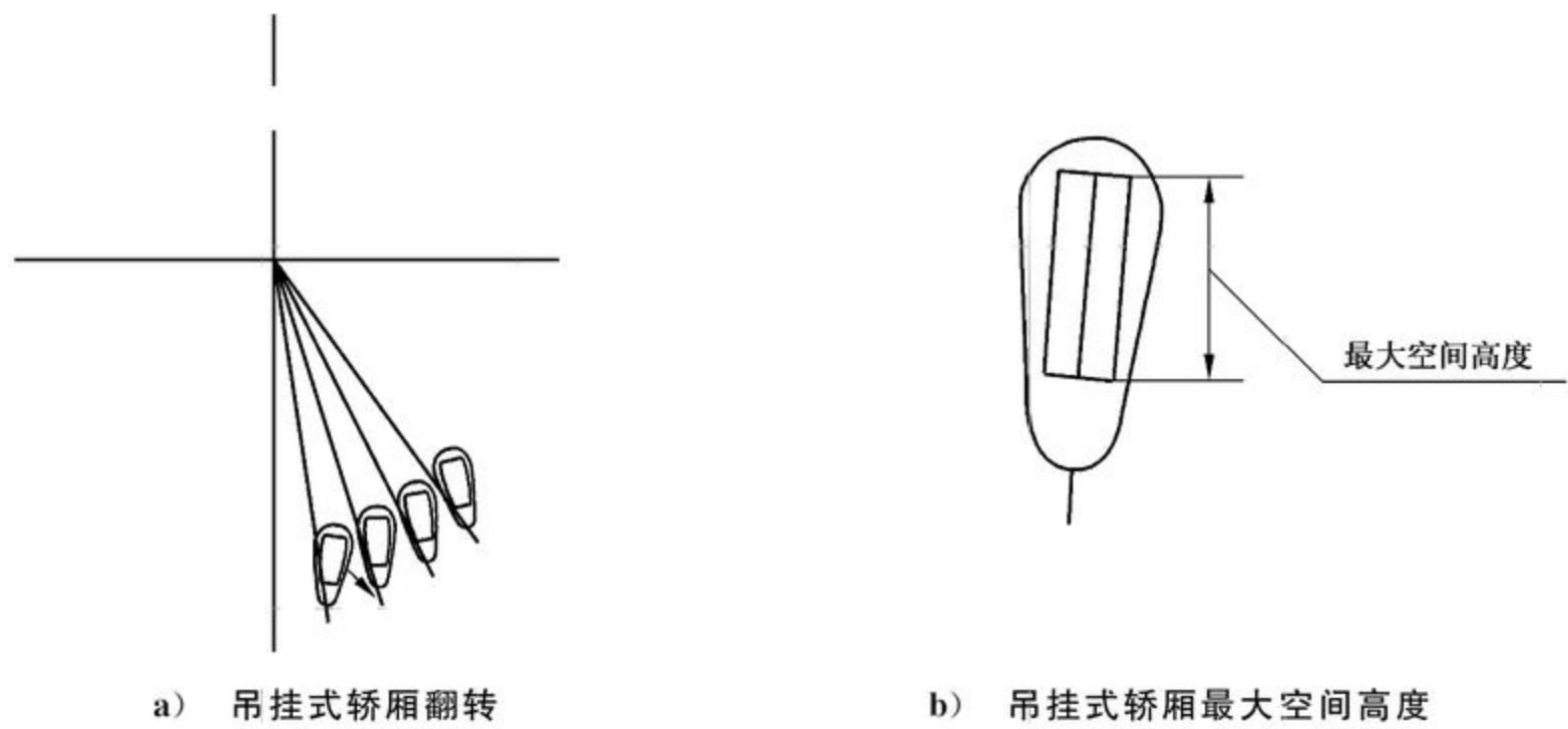
图 C.1 轿厢最大空间高度示意图
