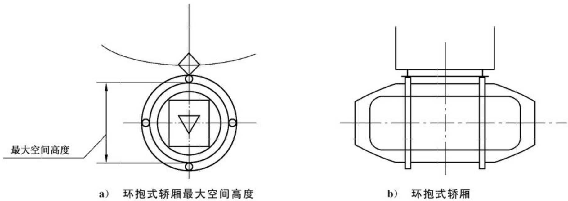
图 C.2 回转式轿厢放大示意图
