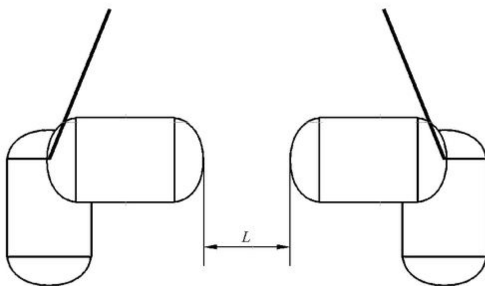
图 C.4 轿厢翻转时需留有距离 L 示意图
