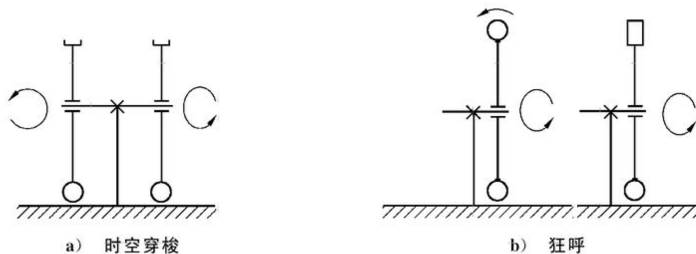
图 A.5 时空穿梭型(E 型)
