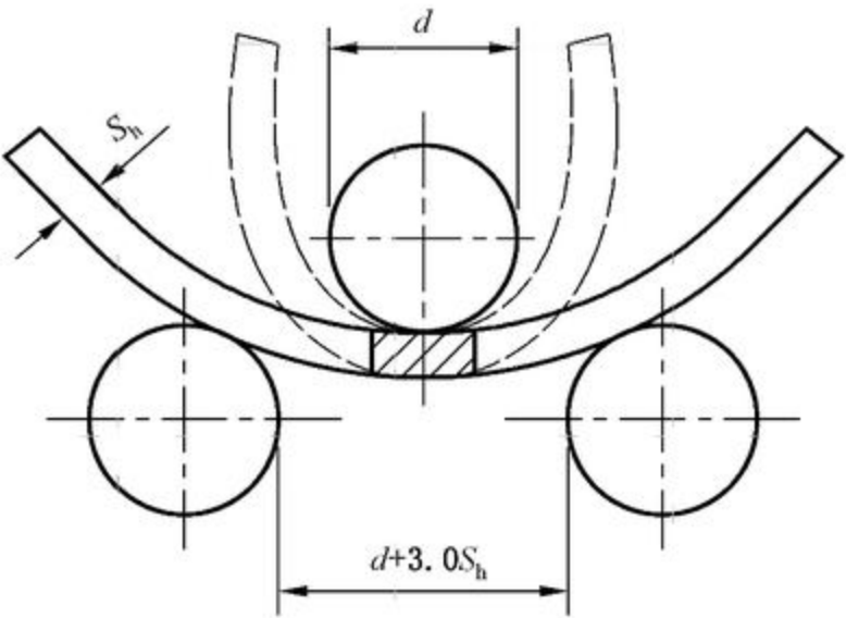
图 11 焊缝接头弯曲试验
