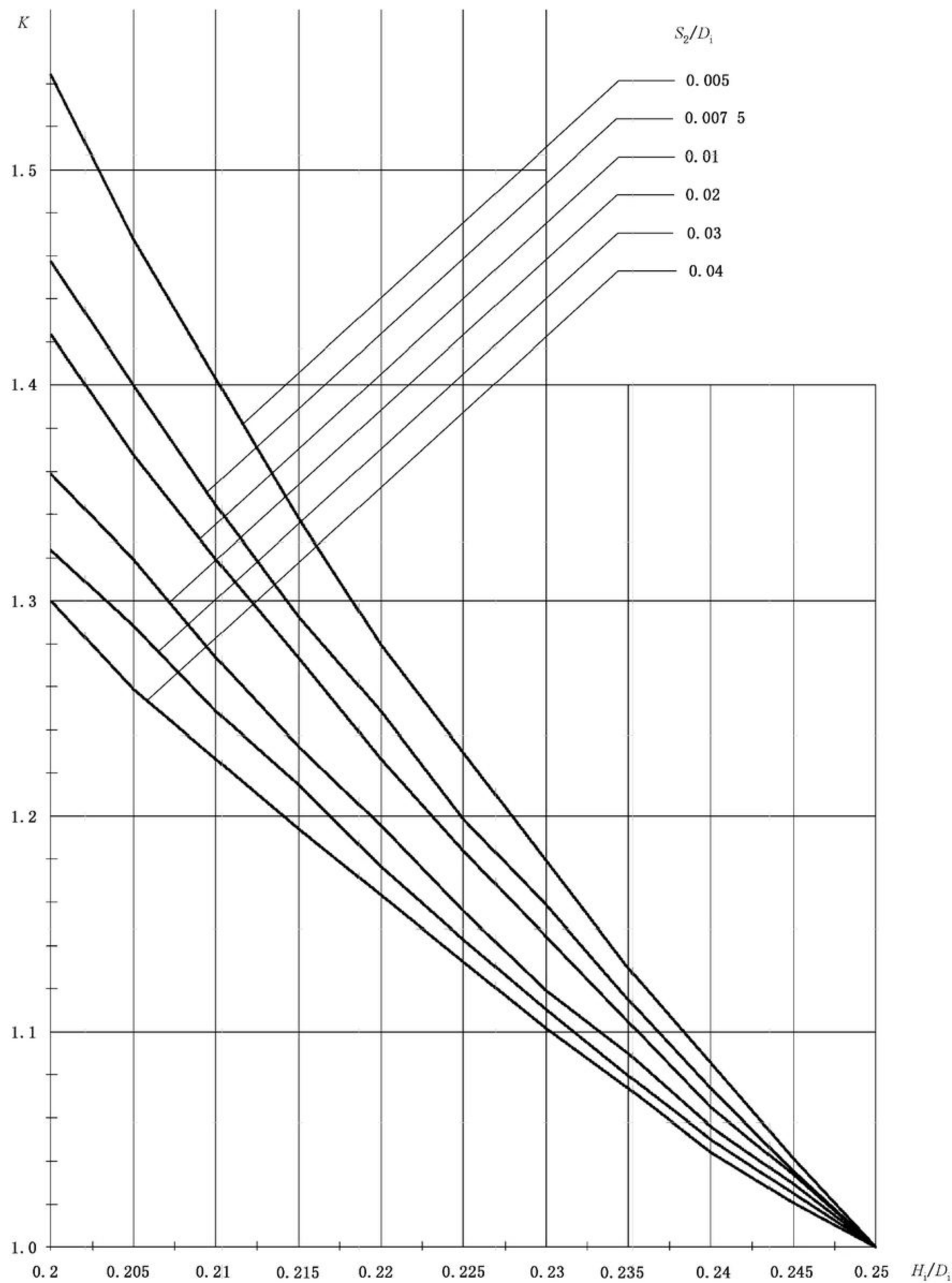
图 4 H_1/D_1 在 0.2~0.25 时的封头形状系数 K
