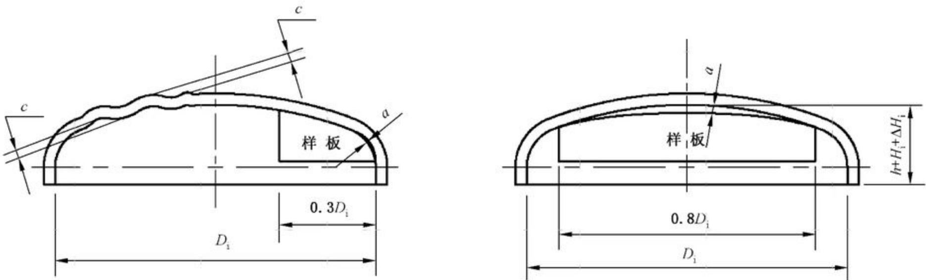
图 6 封头形状与尺寸检查
