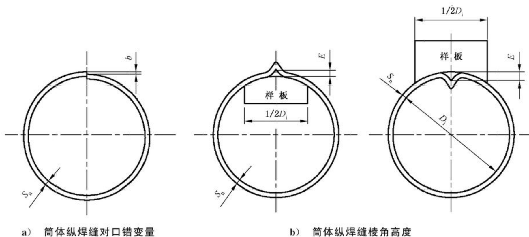
图 7 筒体纵焊缝焊接尺寸检查
