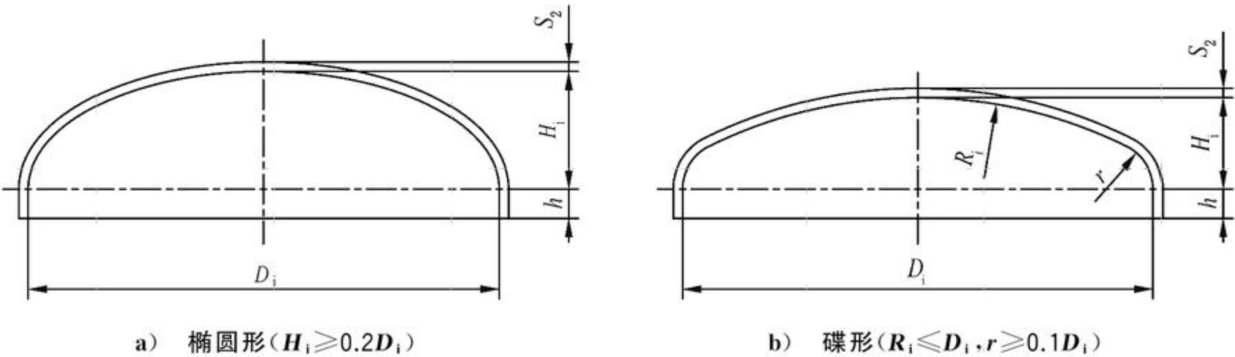
图 3 封头形状
