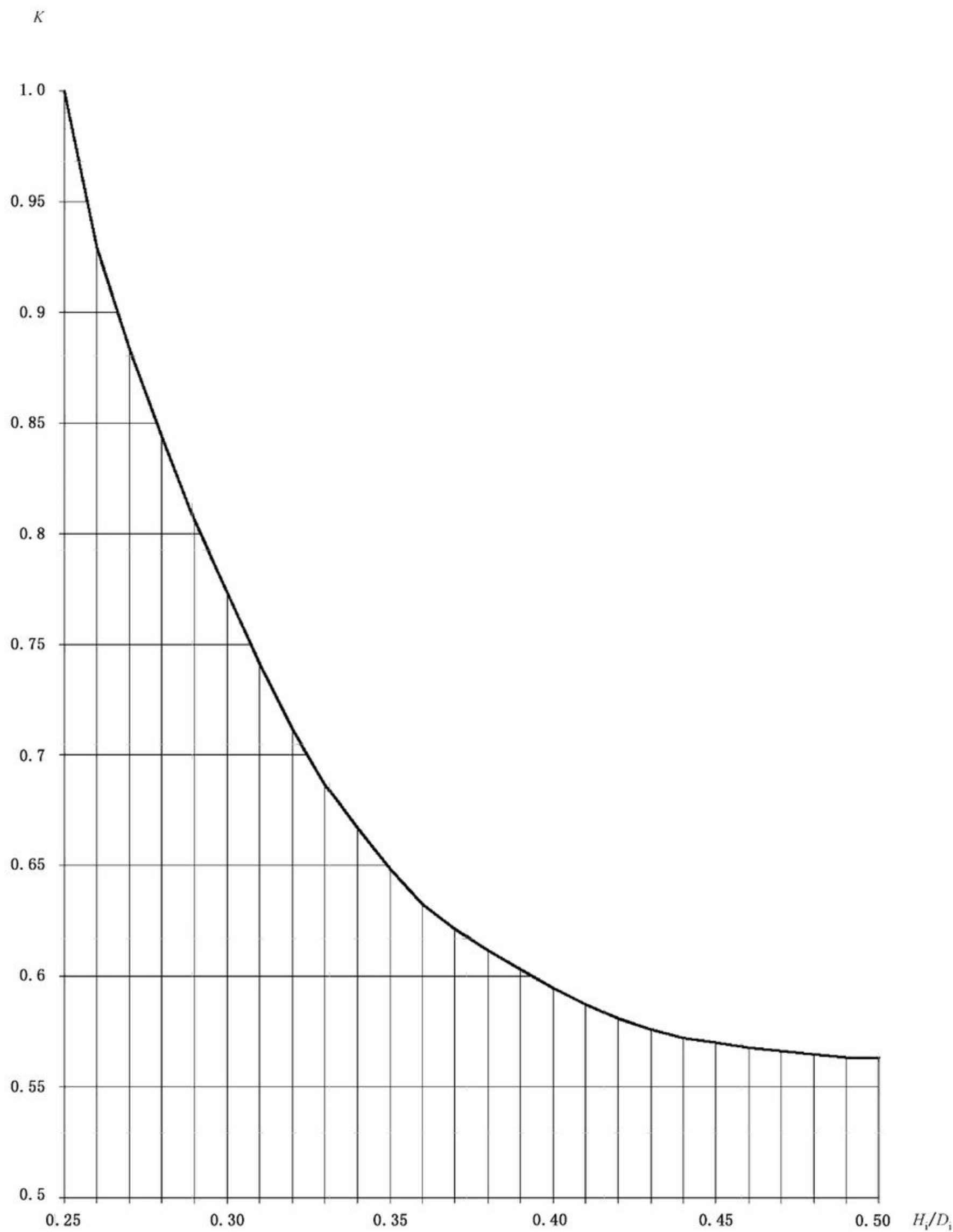
图 5 H_i/D_i 在 0.25~0.50 时的封头形状系数 K
